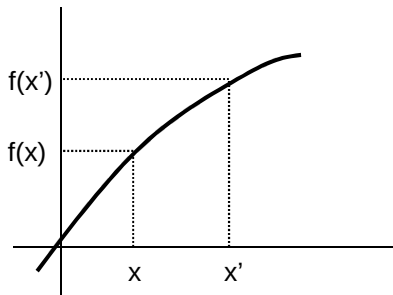
FUNCIÓN CRECIENTE
