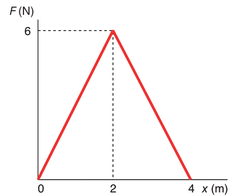
Fig. 7.27. Gráfica fuerza frente a desplazamiento.
