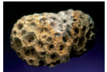
En este fósil de coral cementado, ha precipitado calcita en los huecos que antes ocupaban los pólipos.
