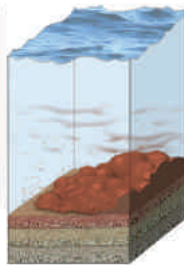
Acreción cinética
