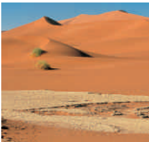
El viento produce una intensa selección de los clastos que transporta. Los granos de arena que forman una duna son todos del mismo tamaño.
