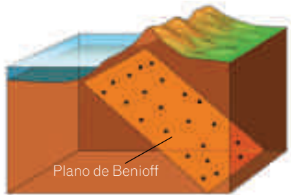
En algunos márgenes continentales los terremotos se disponen sobre un plano inclinado.
