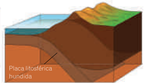
Interpretación de la tectónica de placas: el plano de Benioff es una zona de destrucción de litosfera oceánica.
