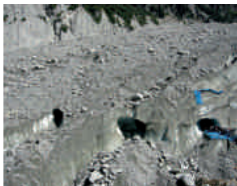
Entradas a grutas excavadas en el hielo del glaciar La Mer de Glace, en los Alpes franceses.
