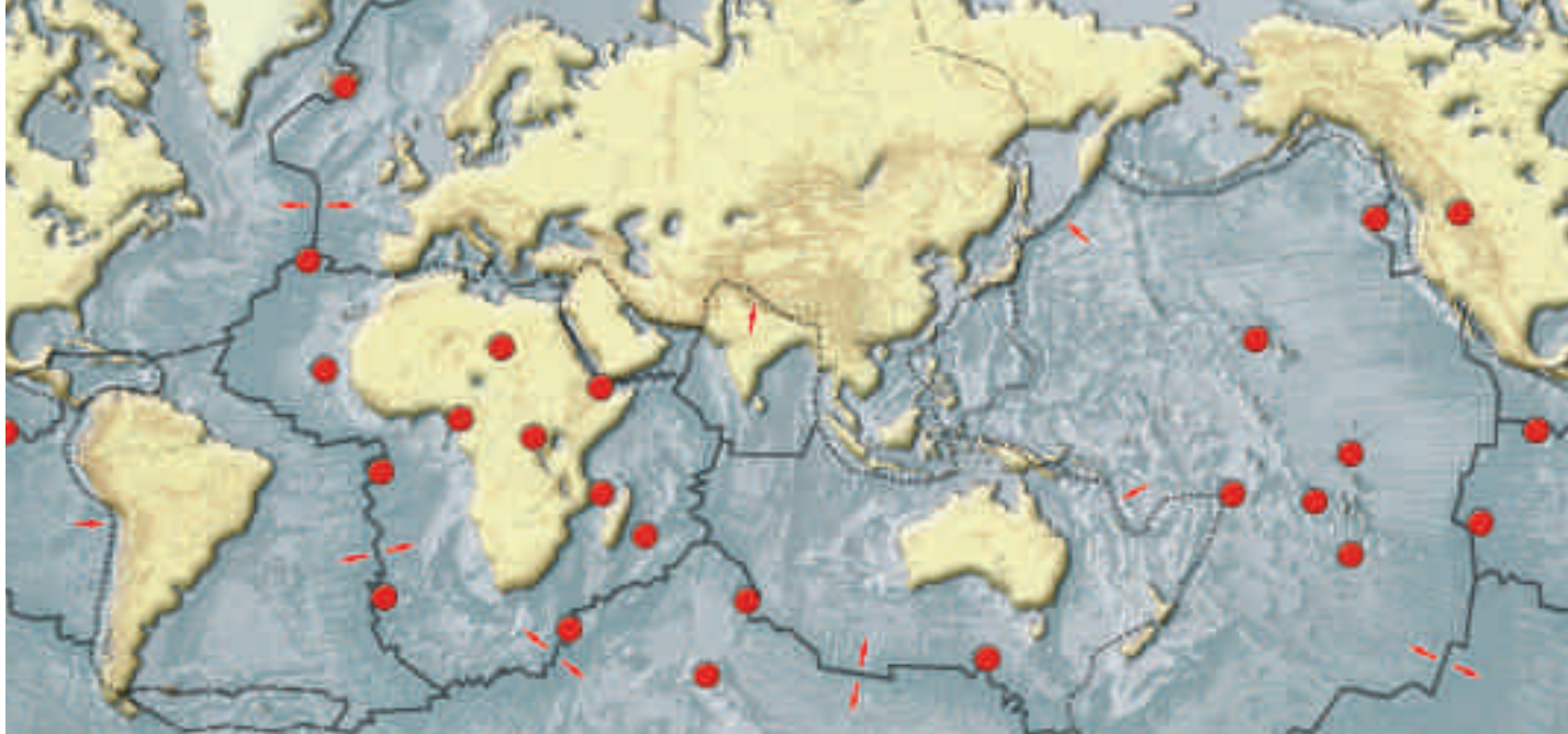
Mapa del relieve de fondos oceánicos. Los puntos rojos corresponden a la situación actual de los principales puntos calientes del planeta. Estudios recientes, publicados en marzo de 2008, parecen demostrar que la localización de los puntos calientes varía con el tiempo, debido a que las corrientes de convección del manto mecen los penachos térmicos desde su base.
