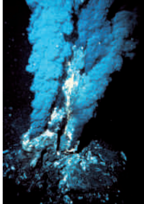
En las dorsales oceánicas siguen viviendo bacterias descendientes de las primeras formas de vida.
