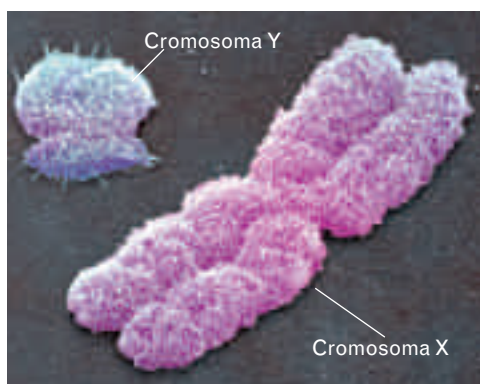
Heterocromosomas.
