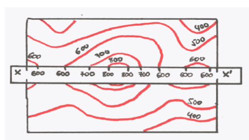
2. SEÑALAR EN UNA TIRA LAS CURVAS DE NIVEL
