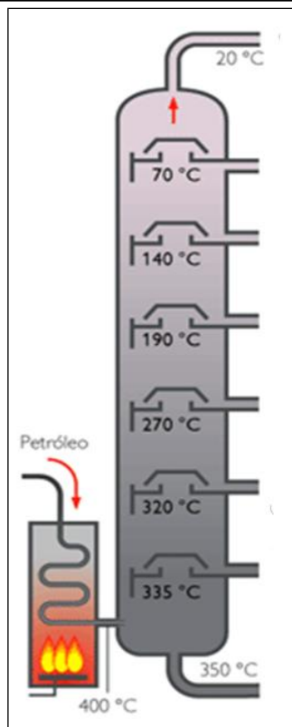
Destilación fraccionada del petróleo. Torre de
