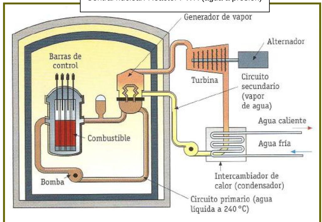
Central nuclear. Reactor PWR (agua a presión)
