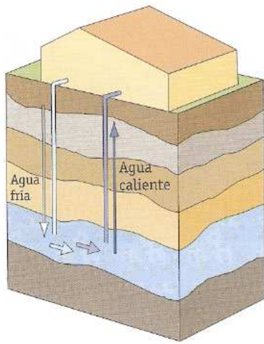
Obtención de energía geotérmica
