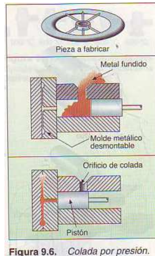
Figura 9.6. Colada por presión.
