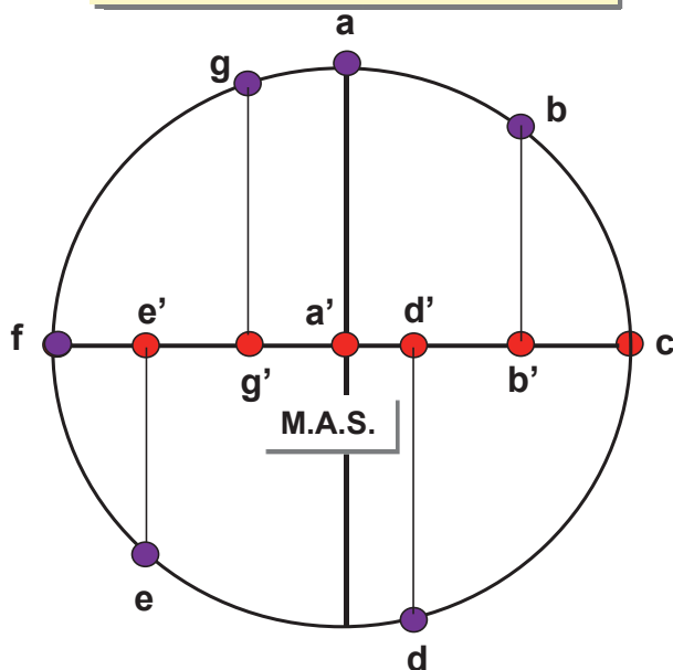
Proyección de un MCU sobre el diámetro de su circunferencia
