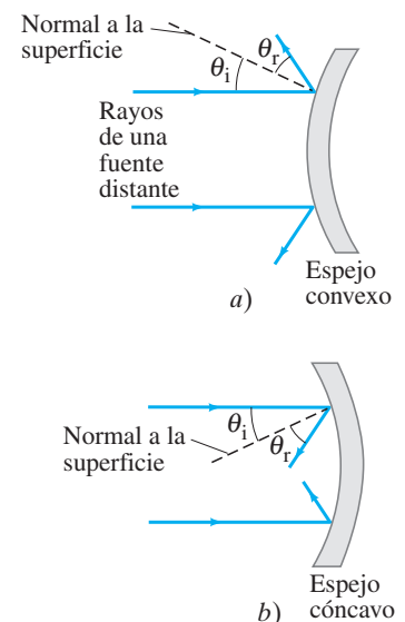
FIGURA 8-8 Espejos con superficies esféricas convexas y cóncavas. Note que \theta_r = \theta_i para cada rayo.
