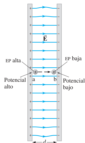
FIGURA 2-1 Al mover la carga positiva de la posición a a la posición b , el campo eléctrico realiza trabajo.
