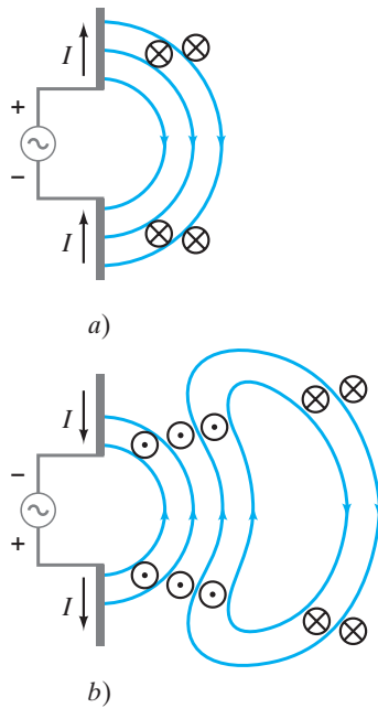
FIGURA 7-5 Secuencia que muestra los campos eléctrico y magnético que se dispersan hacia fuera a partir de cargas en oscilación sobre dos conductores (la antena) conectados a una fuente ca (véase el texto).
