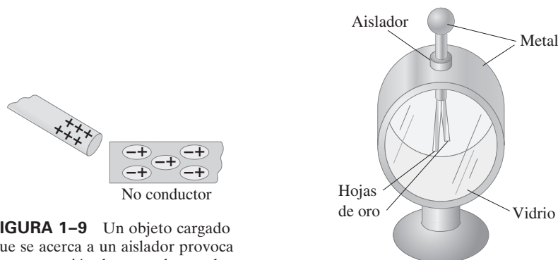
FIGURA 1-10 Electroscopio.
