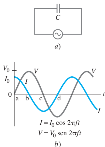
FIGURA 6-37 a ) Capacitor conectado a una fuente ca. b ) La corriente adelanta al voltaje por un cuarto de ciclo, o 90^\circ .
