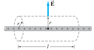
FIGURA 1-40 Cálculo de \vec{E} debido a una línea de carga muy larga, ejercicio H, donde el cilindro que se representa (punteado) es la superficie gaussiana.
