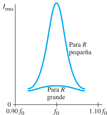
FIGURA 6-42 Corriente en un circuito LRC como función de la frecuencia, que muestra pico de resonancia en f = f_0 = (1/2\pi)\sqrt{1/LC} .
