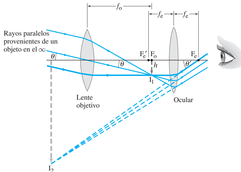
FIGURA 9-19 Telescopio astronómico (refractor). La luz paralela proveniente de un punto sobre un objeto distante ( d_o = \infty ) se lleva a un foco por el lente objetivo en su plano focal. Esta imagen ( I_1 ) se amplifica en el ocular para formar la imagen final I_2 . Sólo dos de los rayos mostrados que entran al objetivo son rayos estándar (2 y 3), como se describió en la figura 8-34.
