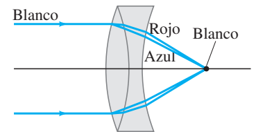
FIGURA 9-27 Doblete acromático.
