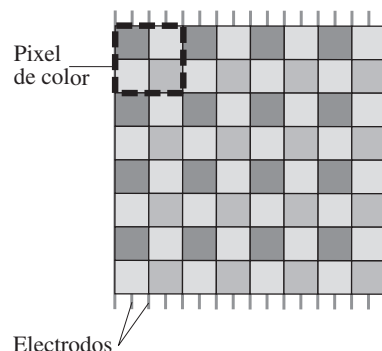
FIGURA 9-2 Porción de un sensor CCD típico. Un grupo cuadrado de cuatro pixeles R_V a veces se llama “pixel de color”.
