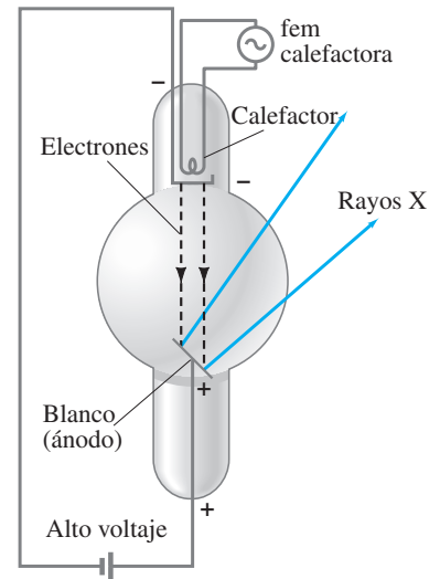
FIGURA 9-35 Tubo de rayos X. Los electrones emitidos por un filamento caliente en un tubo al vacío se aceleran mediante un alto voltaje. Cuando golpean la superficie del ánodo, el “blanco”, se emiten rayos X.
