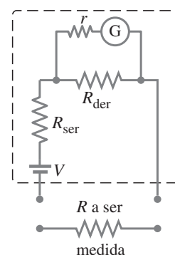
FIGURA 4-32 Un óhmmetro.
