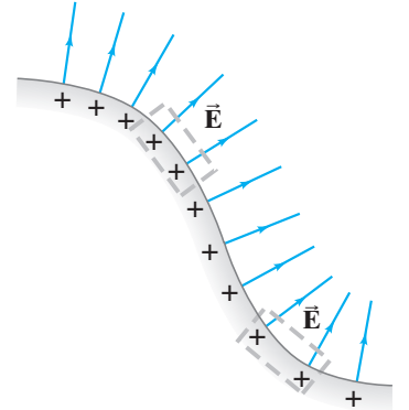
FIGURA 1-41 Campo eléctrico cerca de la superficie de un conductor. Dos pequeñas cajas cilíndricas se indican punteadas. Cualquiera puede servir como la superficie gaussiana. Ejemplo 1-12 .
