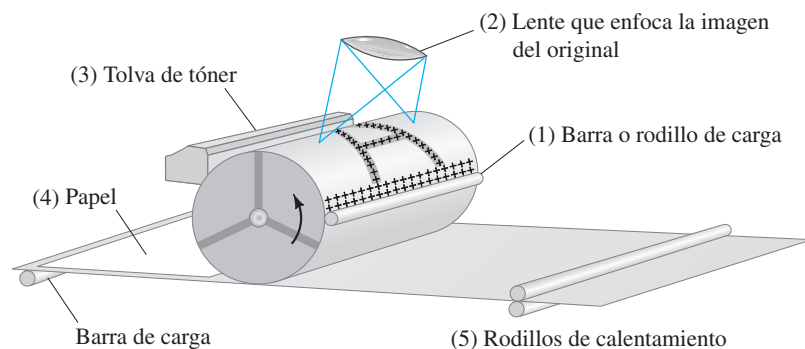
FIGURA 1-46 Interior de una fotocopiadora: 1. al tambor de selenio se le da una carga +; 2. los lentes enfocan la imagen sobre el tambor: sólo los puntos oscuros permanecen cargados; 3. las partículas de tóner (cargadas negativamente) son atraídas hacia las áreas positivas del tambor; 4. la imagen se transfiere al papel; 5. el calor fija la imagen al papel.
