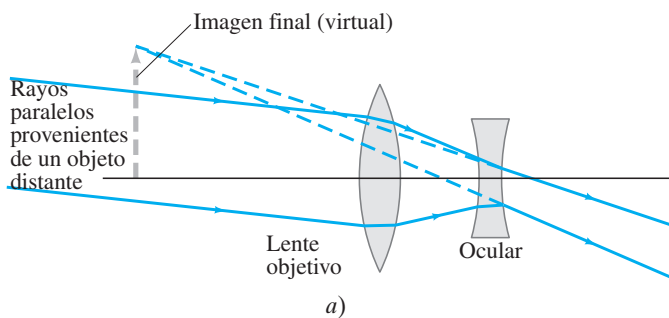
FIGURA 9-22 Telescopios terrestres que producen una imagen derecha: a) galileano; b) tipo catalejo o lente de campo.
