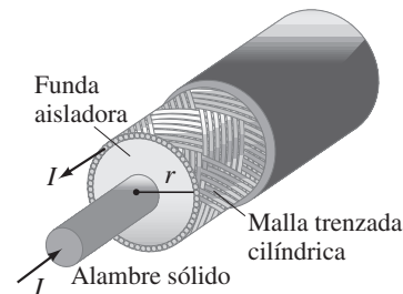
FIGURA 5-63 Cable coaxial. Problema 53.
