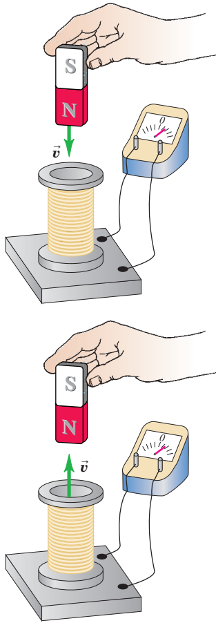
10.1 Se induce la misma fem en la bobina ya sea que (a) el imán se mueva respecto a la bobina o (b) la bobina se mueva respecto al imán.
