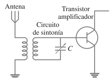
FIGURA 7-16 Sintonización simple de una estación de radio.
