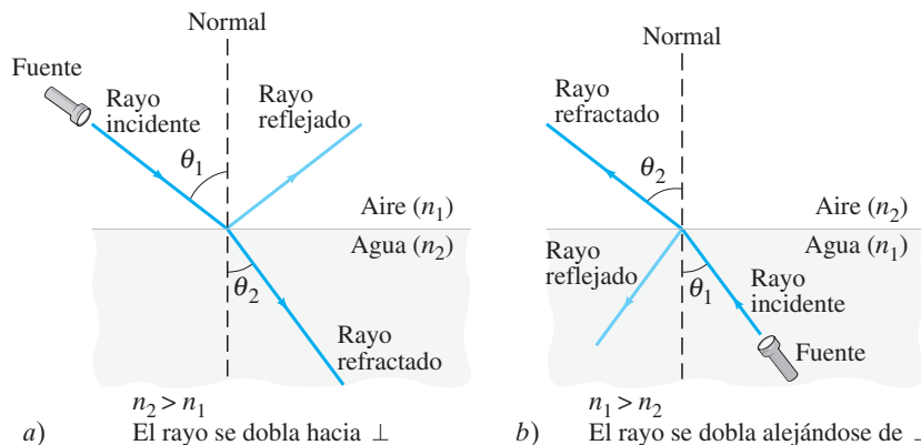
FIGURA 8-19 Refracción. a) Luz refractada cuando pasa del aire ( n_1 ) al agua ( n_2 ): n_2 > n_1 . b) Luz refractada cuando pasa del agua ( n_1 ) al aire ( n_2 ): n_1 > n_2 .
