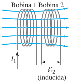
FIGURA 6-31 Una corriente variable en una bobina inducirá una corriente en la segunda bobina.
