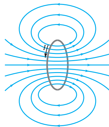
FIGURA 5-9 Líneas de campo magnético debidas a un lazo circular de alambre.
