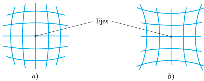
FIGURA 9-25 Distorsión: las lentes forman la imagen de una rejilla cuadriculada de líneas perpendiculares para producir a ) distorsión en barril o b ) distorsión en cojín. Estas distorsiones se aprecian en la fotografía de la figura 8-29d .
