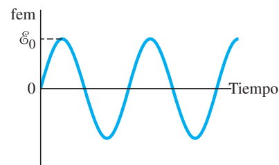
FIGURA 6-18 Un generador ca produce una corriente alterna. La fem de salida \mathcal{E} = \mathcal{E}_0 \sin \omega t , donde \mathcal{E}_0 = N\omega B (ecuación 6-5).
