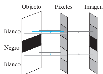
FIGURA 9-3 Suponga que se toma una fotografía que incluye una delgada línea negra (el objeto) sobre un fondo blanco. La imagen de esta línea blanca tiene un halo colorido (rojo arriba, azul abajo) debido al ordenamiento en mosaico de los pixeles de filtro de color, como lo muestran los otros colores transmitidos. El promedio de la computadora permite minimizar los problemas de color como éste (el verde en la parte superior e inferior de la imagen se promedia con los pixeles cercanos para dar blanco o casi blanco), pero la imagen, en consecuencia, se “suaviza” o se vuelve borrosa. Los pixeles de color en capa descritos en el texto evitarían este artefacto.
