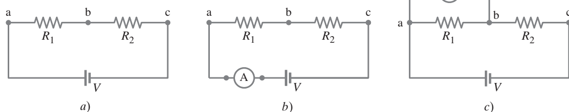
FIGURA 4-33 Medición de corriente y voltaje.
