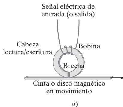
FIGURA 6-27 a) Cabeza de lectura/escritura (reproducción/grabación) para cinta o disco. En la escritura o grabación, la señal eléctrica de entrada hacia la cabeza, que actúa como un electroimán, magnetiza la cinta o disco que pasa. En la lectura o reproducción, el campo magnético variable de la cinta o disco que pasa induce un campo magnético variable en la cabeza, que a su vez induce una fem en la bobina, que es la señal de salida. b) Fotografía de un disco duro que incluye varias placas y cabezas de lectura/escritura que se pueden mover rápidamente del borde del disco hacia el centro.
