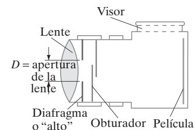
FIGURA 9-1 Una cámara simple.
