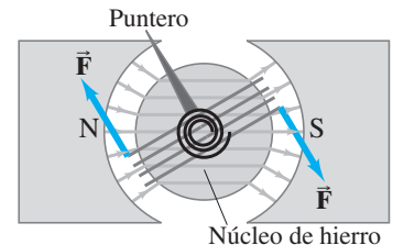
FIGURA 5-34 Bobina de galvanómetro enrollada en un núcleo de hierro.
