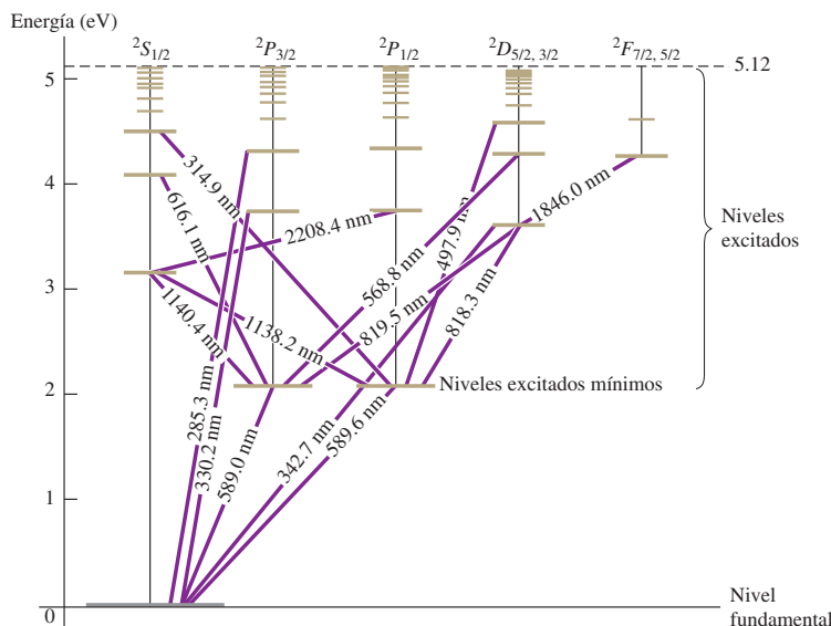
11.10 Niveles de energía del átomo de sodio, en relación con el nivel fundamental. Los números en las líneas que unen los niveles son longitudes de onda. Los encabezados de columna, como 2S_{1/2} , representan algunos estados cuánticos del electrón de valencia.
