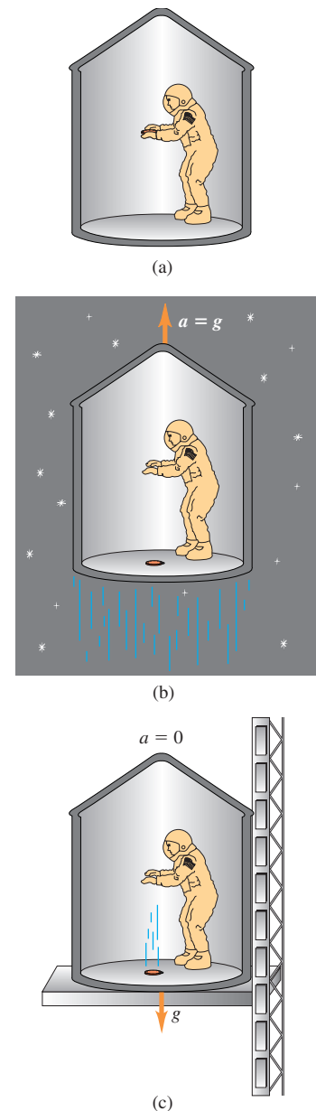
10.21 (a) Un astronauta deja caer su reloj en la nave espacial. (b) En el espacio sin gravedad el piso se acelera hacia arriba a a = g y golpea el reloj. (c) En la superficie terrestre el reloj se acelera hacia abajo a a = g y golpea el piso. Sin información acerca del exterior de la nave, el astronauta es incapaz de distinguir la situación (b) de la situación (c).
