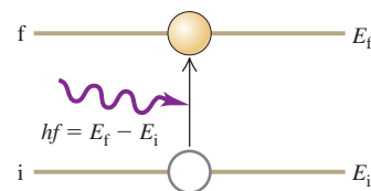
11.11 Un átomo se eleva de un nivel inicial i a un nivel final f , absorbiendo un fotón cuya energía es igual a E_f - E_i . (Compárelo con la Fig. 11.7).
