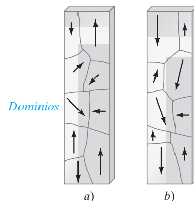
FIGURA 5-40 a) Un pedazo de hierro no magnetizado está constituido por dominios ordenados aleatoriamente. Cada dominio es como un pequeño imán; las flechas representan la dirección de magnetización, siendo la punta de la flecha el polo N. b) En un imán, los dominios están alineados preferentemente en una dirección (hacia abajo en este caso) y se pueden alterar en tamaño por el proceso de magnetización.
