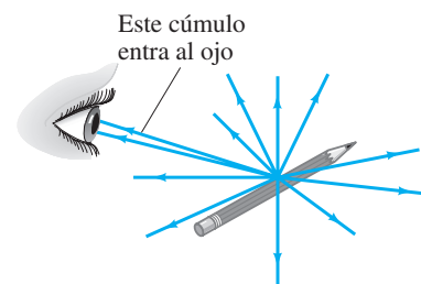
FIGURA 8-1 Los rayos de luz provienen de cada punto individual de un objeto. Se muestra cómo un pequeño cúmulo de rayos que salen de un punto entran a los ojos de una persona.
