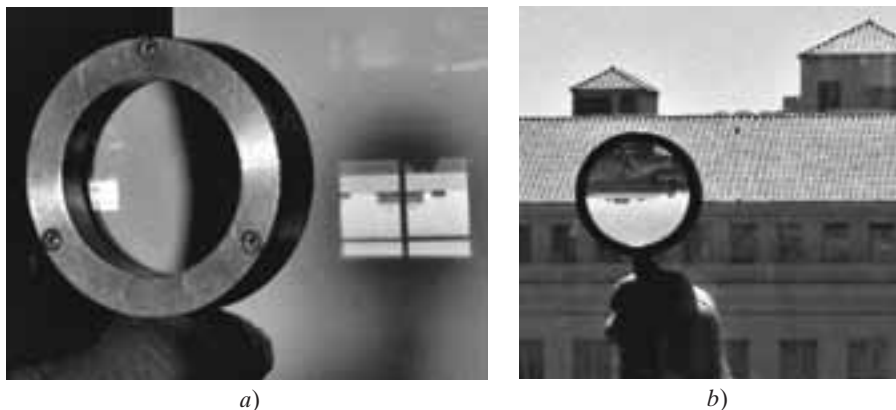
FIGURA 8-35 a) Una lente convergente puede formar una imagen real (aquí de un edificio distante, de cabeza) en una pantalla. b) Esa misma imagen real también es directamente visible al ojo. [La figura 8-29d muestra imágenes (papel gráfico) formadas tanto por lentes divergentes como por convergentes, vistas por el ojo].
