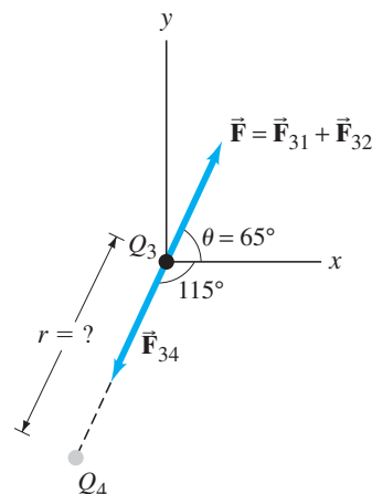
FIGURA 1-21 Ejemplo 1-5 y ejercicio D: Q_4 ejerce una fuerza ( \vec{F}_{34} ) que hace que la fuerza neta sobre Q_3 sea cero.
