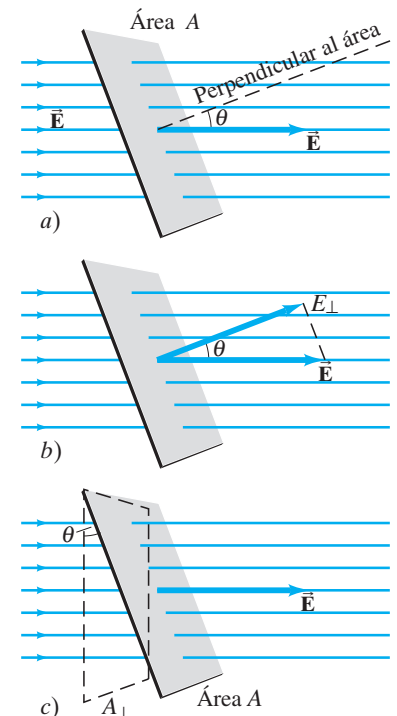
FIGURA 1-37 a) Un campo eléctrico uniforme \vec{E} que pasa a través de una área plana A . b) E_{\perp} = E \cos \theta es el componente de \vec{E} perpendicular al plano de área A . c) A_{\perp} = A \cos \theta es la proyección (punteada) del área A perpendicular al campo \vec{E} .
