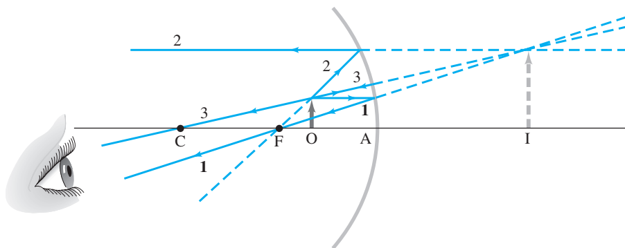
FIGURA 8-16 Objeto colocado dentro del punto focal F. La imagen está detrás del espejo y es virtual , ejemplo 8-3 . [Note que la escala vertical (altura del objeto = 1.0 cm) es diferente de la horizontal (OA = 10.0 cm) para facilitar el dibujo, aunque esto afecta la precisión del mismo].
