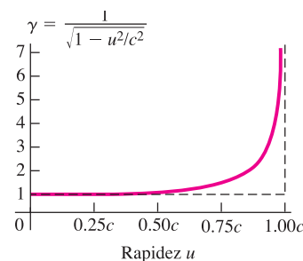
10.7 La cantidad \gamma = 1/\sqrt{1 - u^2/c^2} en función de la rapidez relativa u de dos marcos de referencia.
