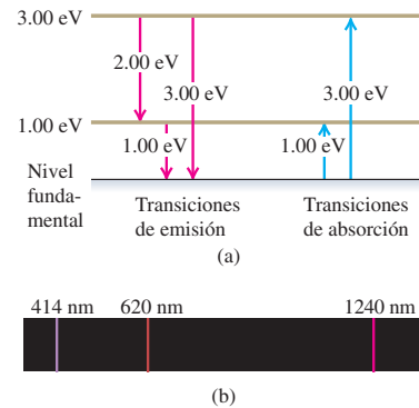
11.13 (a) Diagrama de niveles de energía que muestra las transiciones posibles para emisión desde niveles excitados, y para absorción desde el nivel fundamental. (b) Espectro de emisión de este átomo hipotético.
