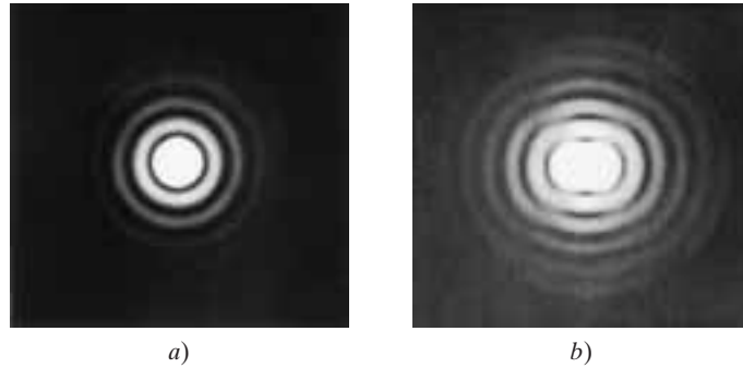
FIGURA 9-28 Fotografías de imágenes (enormemente amplificadas) formadas por una lente, que muestran el patrón de difracción de una imagen para a) un solo objeto puntual, b) dos objetos puntuales cuyas imágenes tienen baja resolución.
