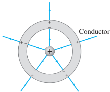
FIGURA 1-33 Una carga dentro de un cascarón metálico esférico neutro induce carga sobre sus superficies. El campo eléctrico existe incluso más allá del cascarón, pero no dentro del conductor mismo.
