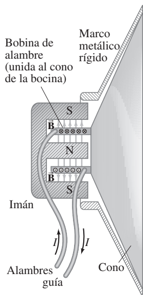
FIGURA 5-38 Bocina.
