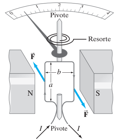
FIGURA 5-33 Galvanómetro.
