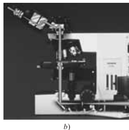
FIGURA 9-23 Microscopio compuesto: a) diagrama de rayos, b) fotografía (la iluminación viene de la esquina inferior derecha, luego sube a través del portaobjetos que sostiene al objeto).
