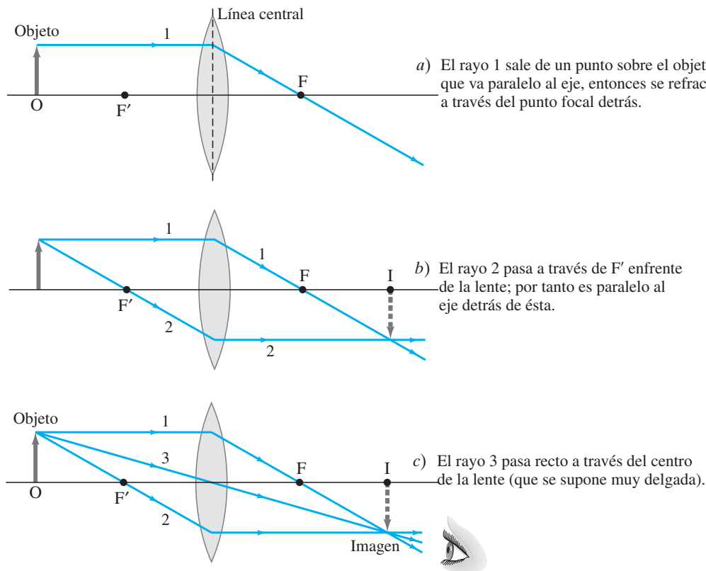
FIGURA 8-34 Cómo encontrar la imagen por trazado de rayos para una lente convergente. Los rayos se muestran saliendo de un punto en el objeto (una flecha). Se ilustran los tres rayos más útiles, que salen de la punta del objeto, para determinar dónde se forma la imagen de ese punto.
