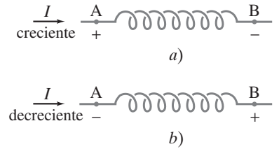
FIGURA 6-32 Ejemplo 6-13. Los signos + y - se refieren a la fem inducida debida a la corriente variable, como si los puntos A y B fuesen las terminales de una batería.
