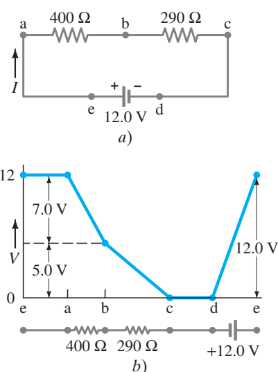
FIGURA 4-12 Los cambios en el potencial alrededor del circuito en a) se grafican en b) .
