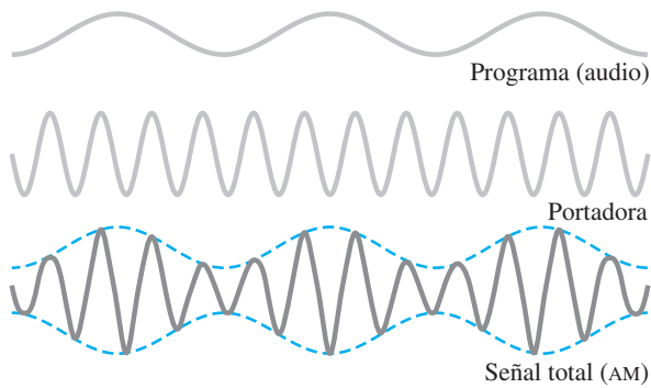
FIGURA 7-13 En amplitud modulada (AM), la amplitud de la señal portadora varía en proporción a la amplitud de la señal de audio.
