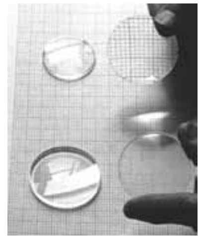
FIGURA 8-29 a) Lentes convergentes y b) lentes divergentes, mostradas en sección transversal. c) Fotografía de una lente convergente (izquierda) y de una lente divergente (derecha). d) Lentes convergentes (arriba) y lentes divergentes (abajo), planas y elevadas sobre el papel para formar imágenes.
