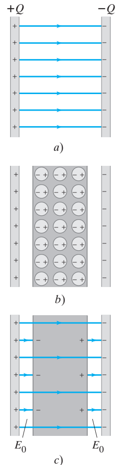
FIGURA 2-16 Vista molecular de los efectos de un dieléctrico.
