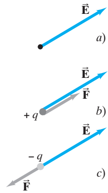
FIGURA 1-24 a) Campo eléctrico en un punto dado en el espacio. b) Fuerza sobre una carga positiva en ese punto. c) Fuerza sobre una carga negativa en ese punto.
