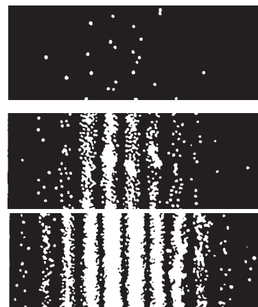
11.33 En estas imágenes se registran las posiciones donde los fotones individuales llegan a la pantalla, en un experimento de interferencia con dos rendijas. La imagen superior muestra la figura después de haber llegado a la pantalla 21 fotones; la de en medio, después de 1000 fotones, y la inferior, después de 10,000 fotones. A medida que llegan más y más fotones a la pantalla, aparece una figura de interferencia reconocible.
