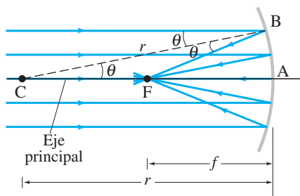
FIGURA 8-12 Los rayos paralelos al eje principal de un espejo esférico cóncavo llegan a un foco en F, el punto focal, siempre que el ancho del espejo sea menor que su radio de curvatura, r , de modo que los rayos son “paraxiales”, es decir, sólo forman ángulos pequeños con el eje.
