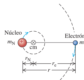
11.20 El núcleo y el electrón giran en torno a su centro de masa común. Se ha exagerado la distancia r_N para tener claridad; para el hidrógeno ordinario, en realidad es igual a r_e/1836.2 .
