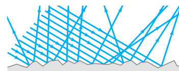
FIGURA 8-3 Reflexión difusa sobre una superficie rugosa.
