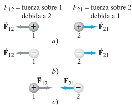
FIGURA 1-15 La dirección de la fuerza depende de si las cargas tienen el mismo signo, como en a) y b), o signos opuestos, como en c).
