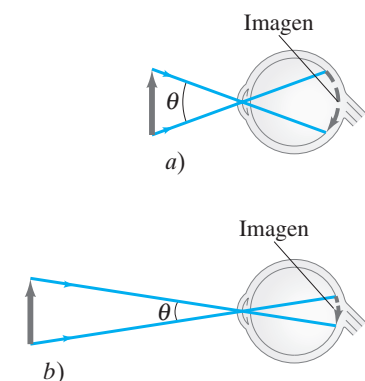
FIGURA 9-15 Cuando el mismo objeto se ve a una distancia más corta, la imagen sobre la retina es más grande, de modo que el objeto parece de mayor tamaño y se distinguen más detalles. El ángulo \theta que el objeto subtiende en a) es más grande que el de b). Nota: Éste no es un diagrama de rayos normal porque sólo se muestra un rayo de cada punto.
