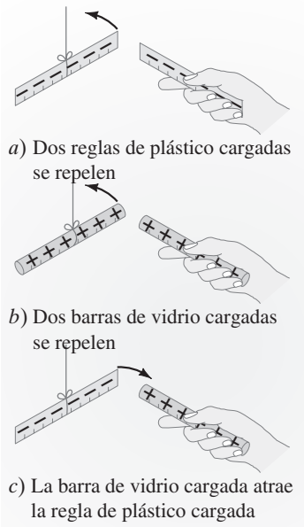
FIGURA 1-2 Cargas iguales se repelen; cargas opuestas se atraen.
