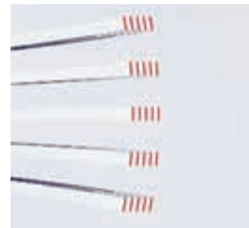
(c) Formación desplazándose hacia la derecha a 0.9c
