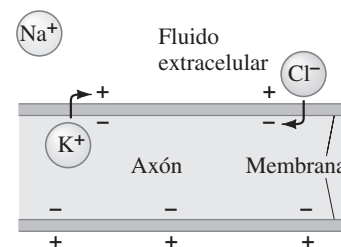
FIGURA 3-28 Cómo se forma una capa dipolo de carga en la membrana de una célula.
