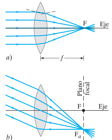
FIGURA 8-31 (abajo) Rayos paralelos llegan a un foco por medio de una lente delgada convergente.
