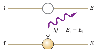
11.7 Un átomo cae de un nivel inicial i a un nivel final de menor energía f, emitiendo un fotón con energía igual a E_i - E_f .
