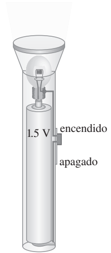
FIGURA 3-10 Linterna (ejemplo 3-3). Aquí se nota cómo el circuito se completa a través de la tira lateral.
