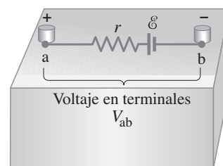
FIGURA 4-1 Diagrama de una pila o batería eléctrica.
