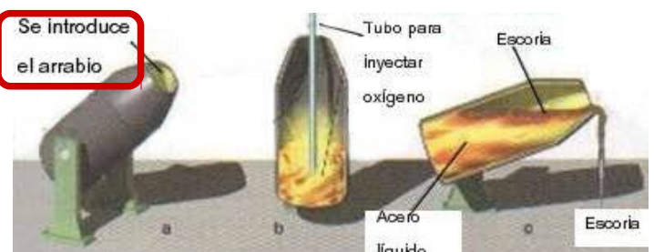
En el convertidor se introduce arrabio para obtener acero
