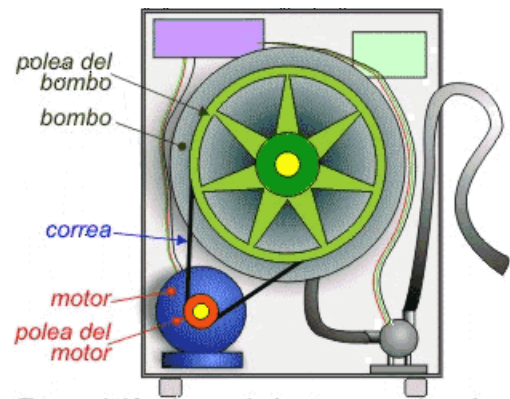
Transmisión de movimiento en una lavadora
