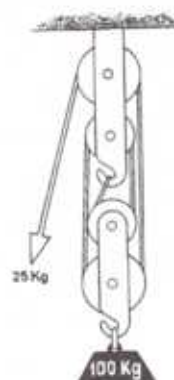
Polipasto
