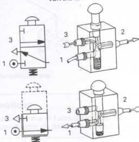
válvula 3/2
