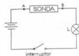
Indicador de humedad
