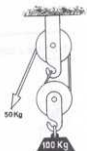
Polipasto
