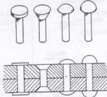
cabeza plana cabeza avellanada cabeza de lenteja cabeza esférica
