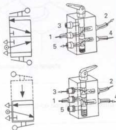
válvula 5/2
