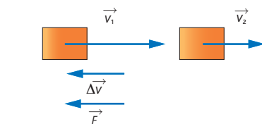
FIGURA 4 Un objeto con trayectoria rectilínea frena disminuyendo el módulo de su velocidad de v_1 a v_2 . El vector \vec{F} tiene la misma orientación que \Delta \vec{v} , y por tanto que \vec{a} (horizontal hacia la izquierda).
