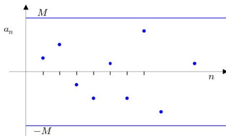
Sucesión acotada |a_n| \leq M
