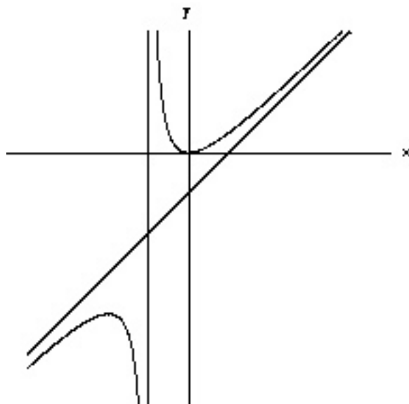
Figura 9.1: La asíntota oblicua es y = x - 1
