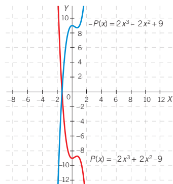
Polinomios opuestos.
