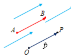
Vector libre \vec{p} . Es equipolente a \overrightarrow{AB} .
