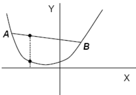
Función convexa
