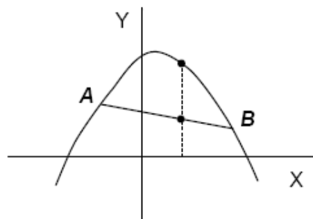
Función cóncava
