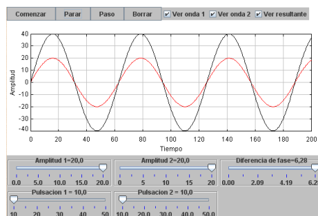
Figura 1.6: Interferencia constructiva
