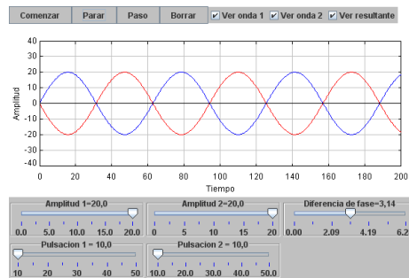
Figura 1.5: Interferencia destructiva
