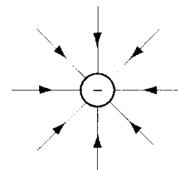
Líneas de campo eléctrico Q -
