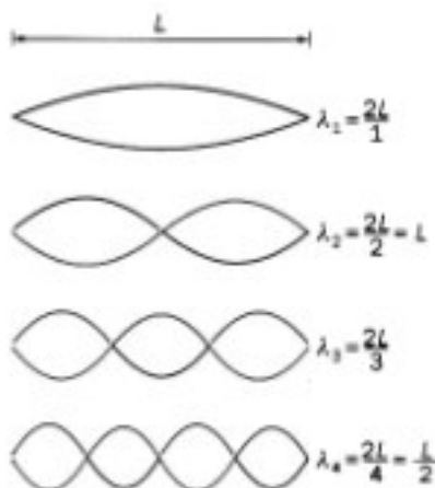
Representación de cuatro modos normales de vibración de una cuerda fija por sus extremos.
