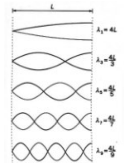
Ondas estacionarias en una cuerda fija por un extremo y libre en el otro
