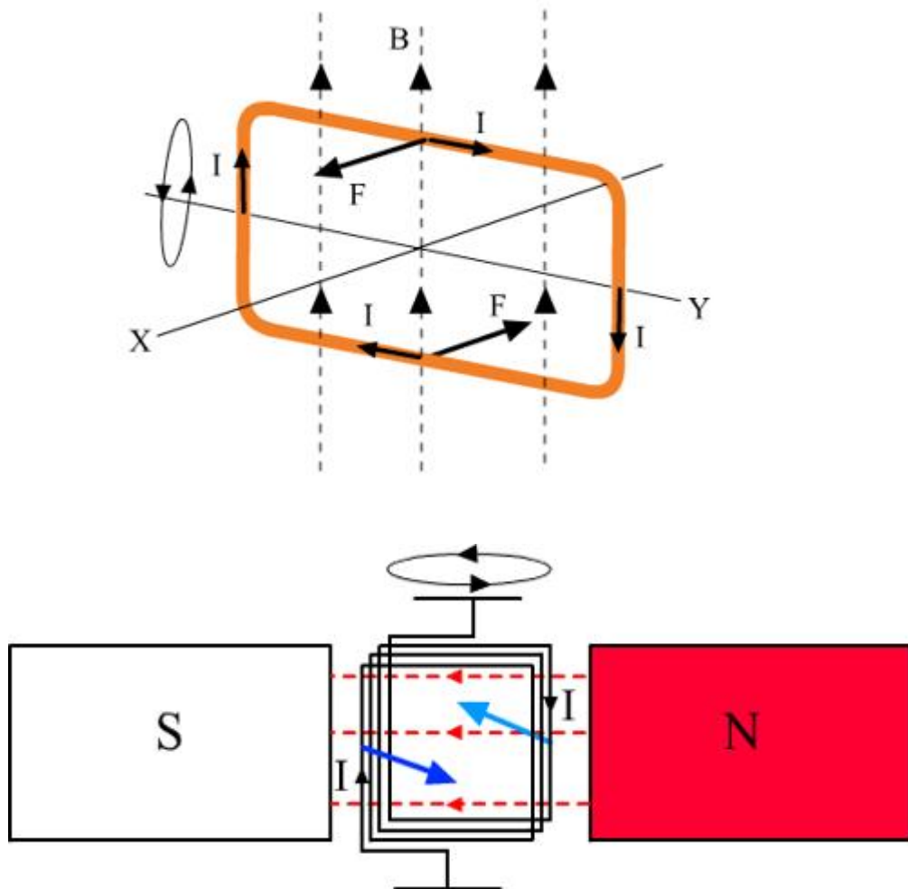
Esquema de un galvanómetro.
