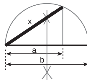
Teorema del cateto
